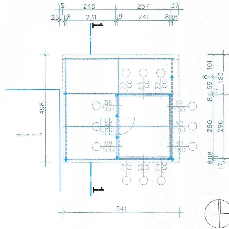
TLOCRT PRIZEMLJA
